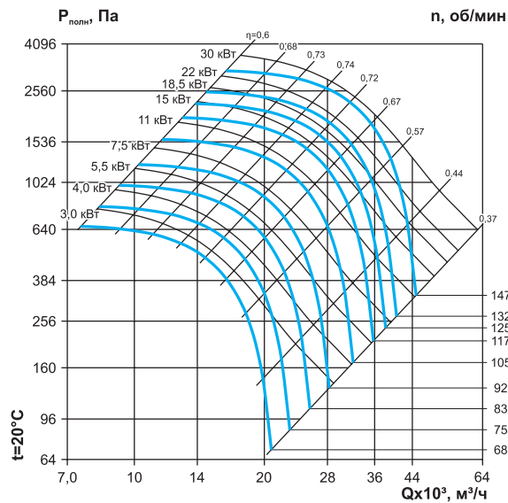
ВР 60-92-9,0 (с частотным регулятором)
