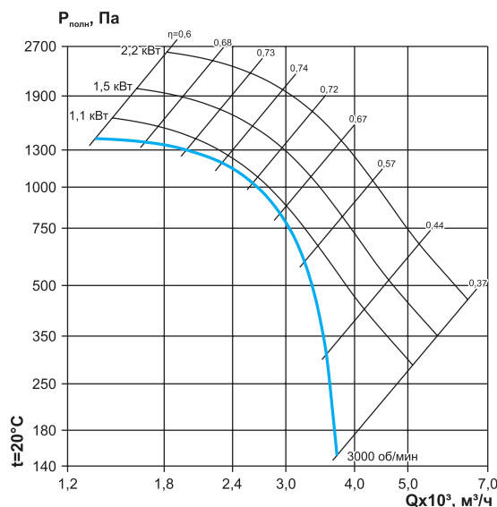
ВР 60-92-3,15 (без частотного регулятора)
