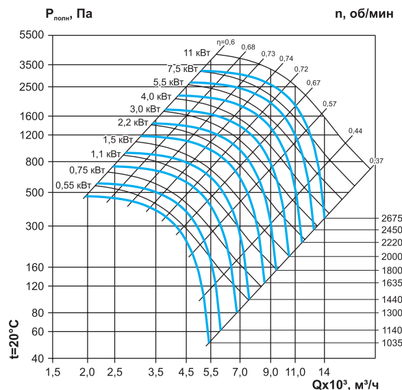
ВР 60-92-5,0 (с частотным регулятором)
