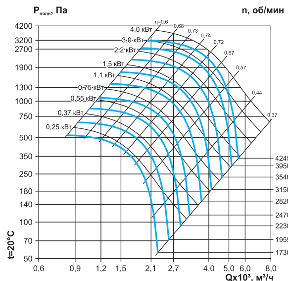
ВР 60-92-3,15 (с частотным регулятором)
