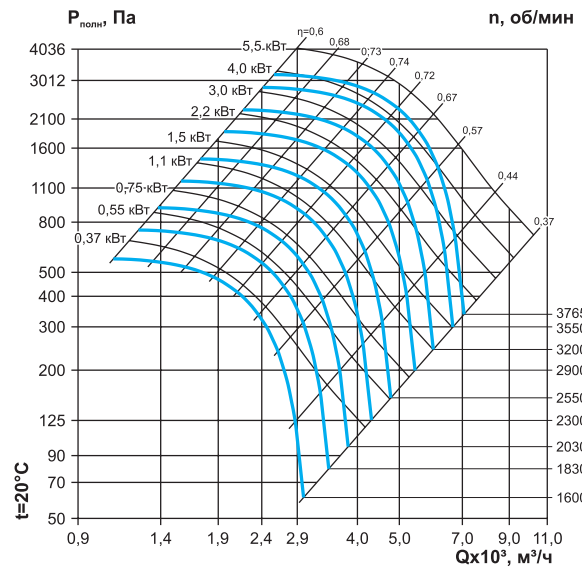
ВР 60-92-3,5 (с частотным регулятором)
