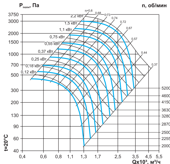
ВР 60-92-2,5 (с частотным регулятором)
