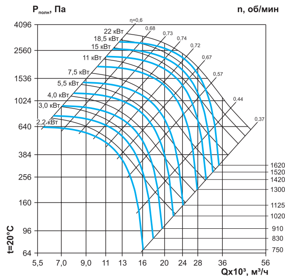
ВР 60-92-8,0 (с частотным регулятором)
