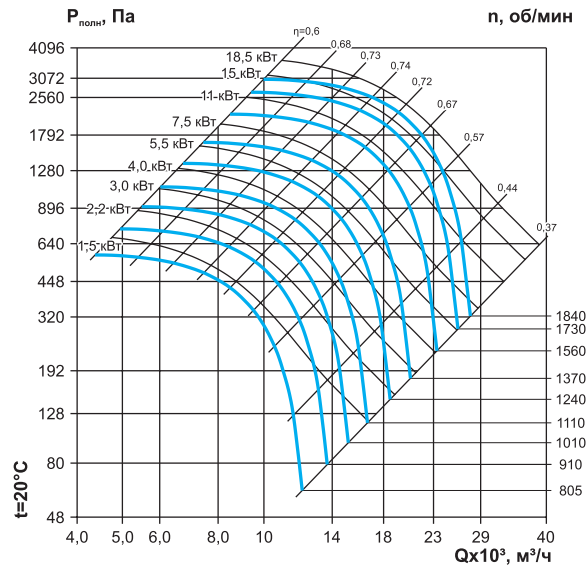
ВР 60-92-7,1 (с частотным регулятором)
