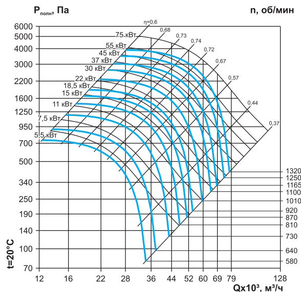
ВР 60-92-11,2 (с частотным регулятором)
