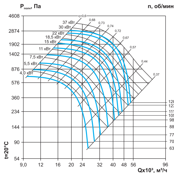
ВР 60-92-10,0 (с частотным регулятором)
