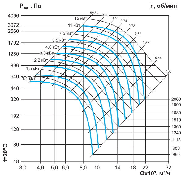
ВР 60-92-6,3 (с частотным регулятором)
