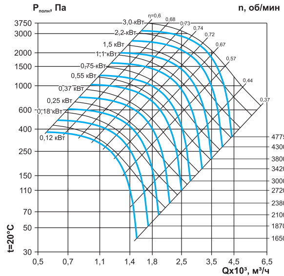
ВР 60-92-2,8 (с частотным регулятором)
