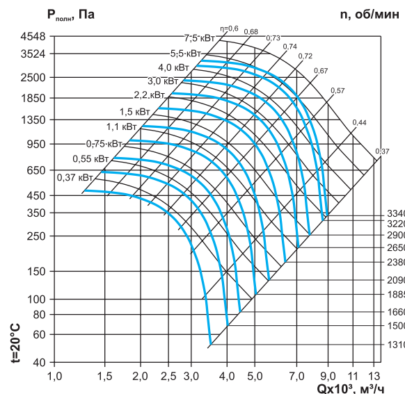
ВР 60-92-4,0 (с частотным регулятором)
