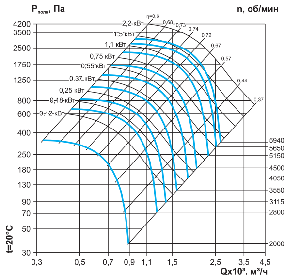
ВР 60-92-2,2 (с частотным регулятором)
