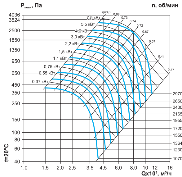
ВР 60-92-4,5 (с частотным регулятором)
