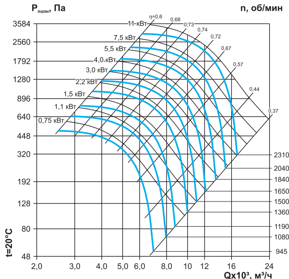
ВР 60-92-5,6 (с частотным регулятором)
